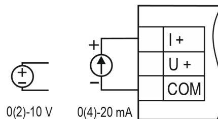
Fig. 5.5 Input wiring
